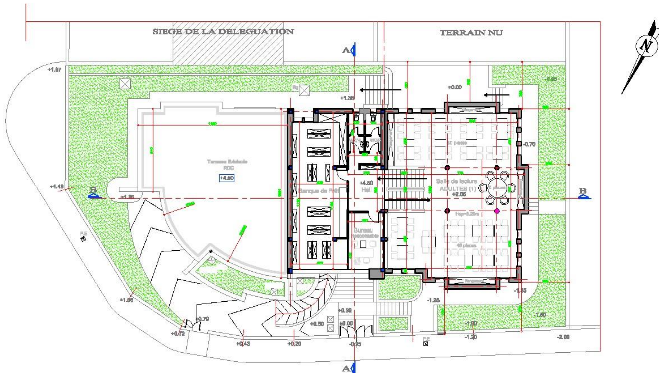
PLAN 2ème NIVEAU +2.85 et +4.50 ECH : 1/100
