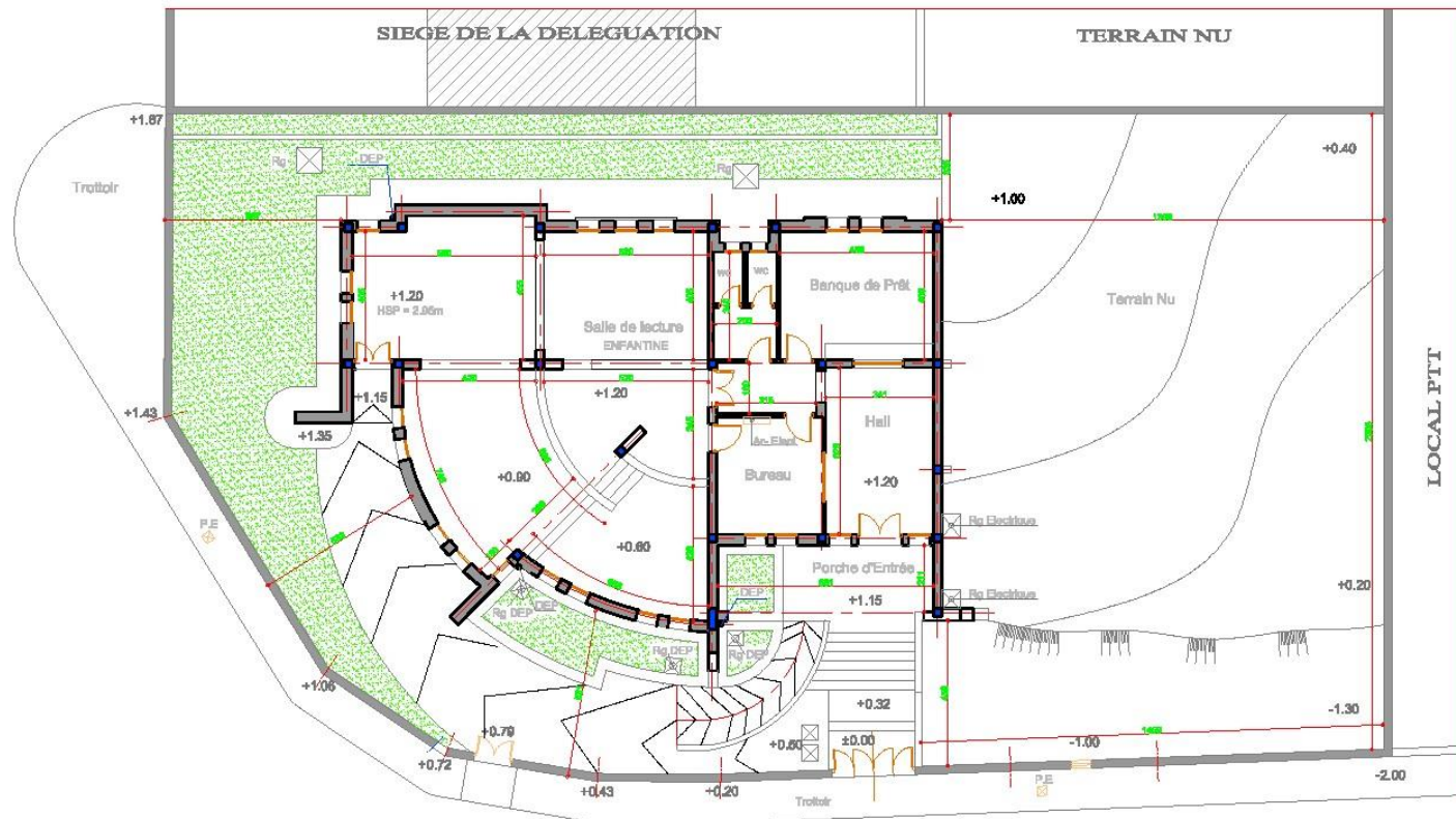
PLAN ETAT EXISTANT ECH 1/100
