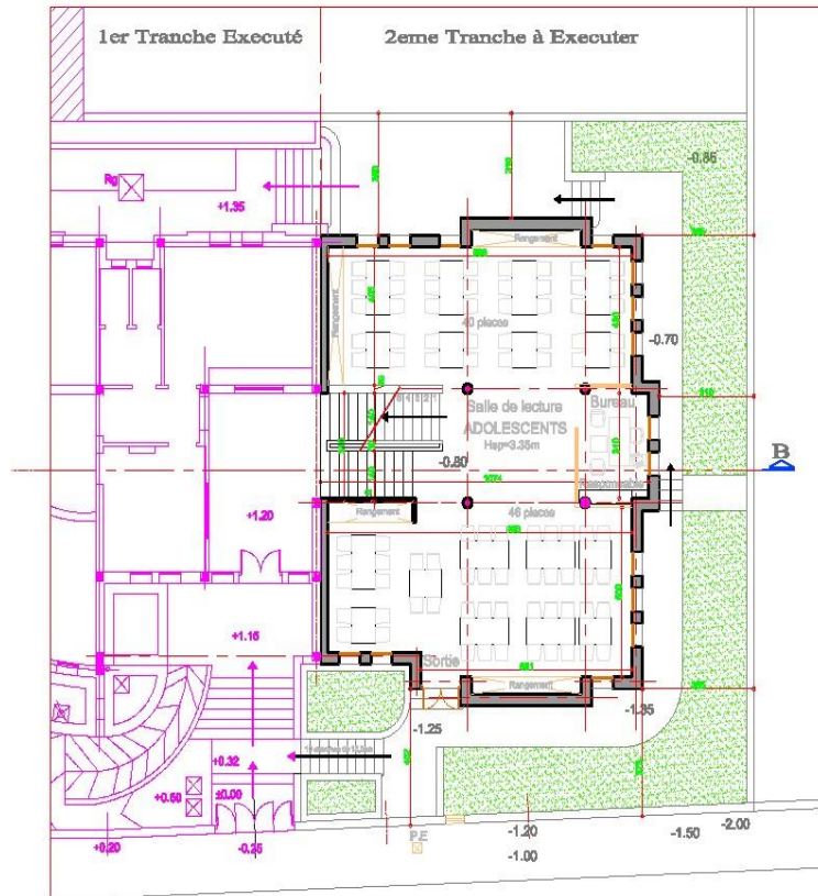
PLAN 1er Niveau -1.10 ECH : 1/100
